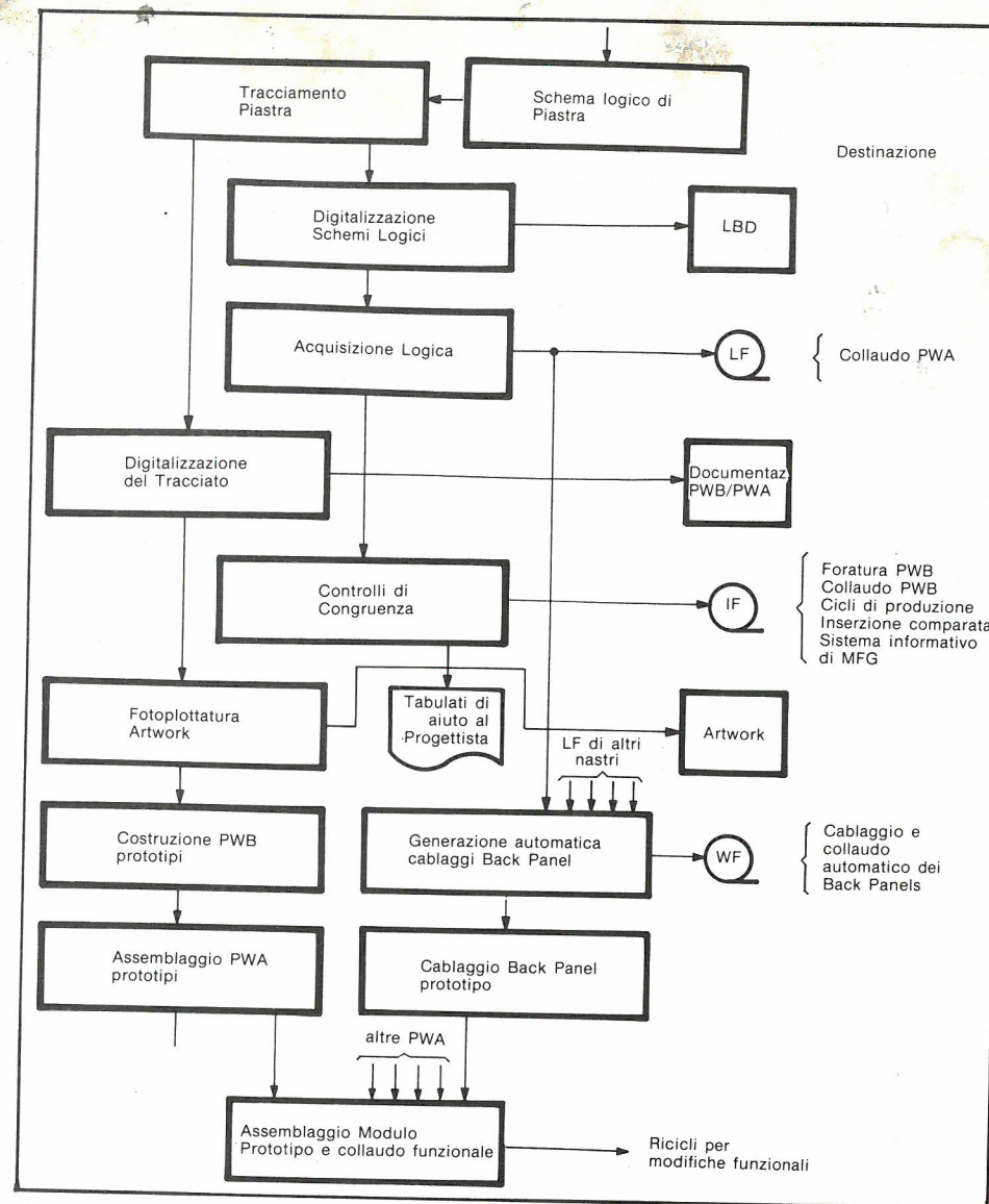
Fig. 2 - Il ciclo tipo che evidenzia i documenti prodotti.
