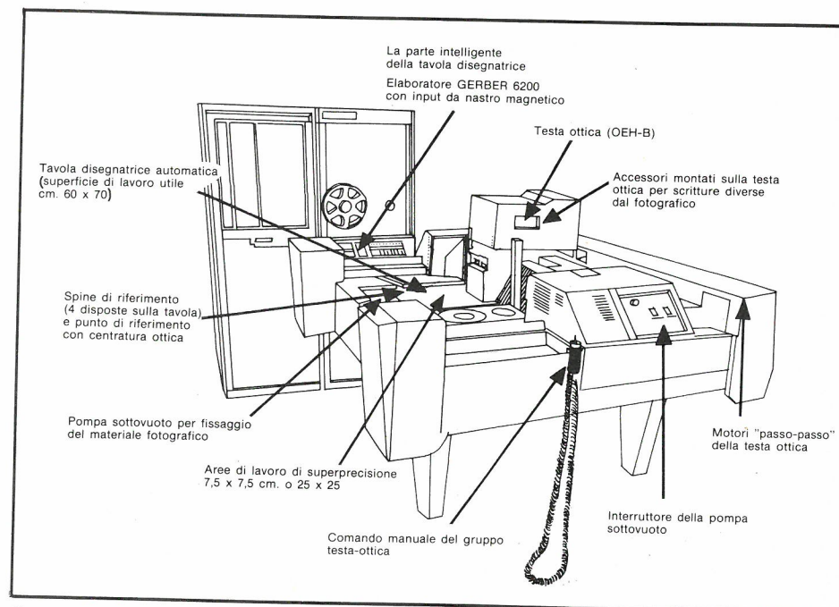
Fig. 3 - L'elaboratore Gerber Model 33 B Photoplotter utilizzato a Pregnana.
